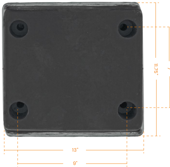
ANCHO Y ALTO DEL TOPE Vista frontal.
